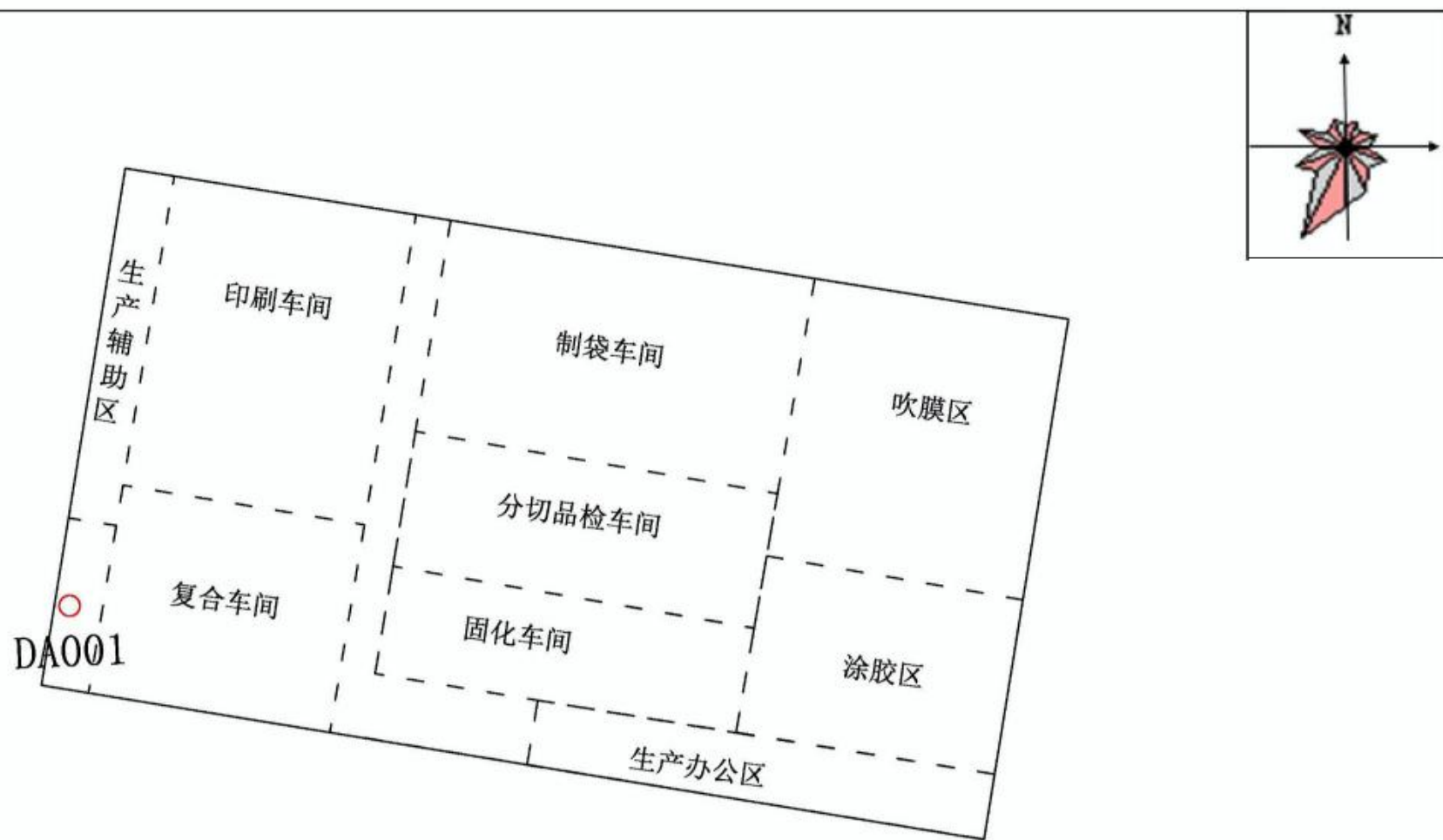
附图3-2 车间内部 平面布置图
