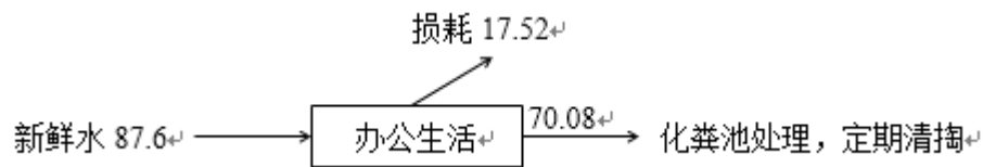
图 2-6 水平衡图 单位：m 3 /d
