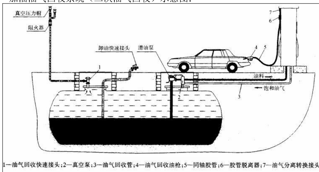
加油油气回收系统（二次油气回收）示意图：
