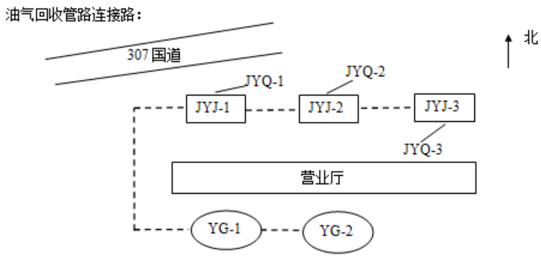
图 6-2 油气回收管路示意图
