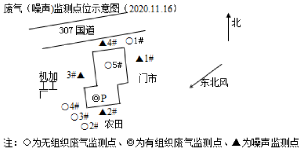
图 6-1 无组织废气及厂界噪声监测点位示意图
